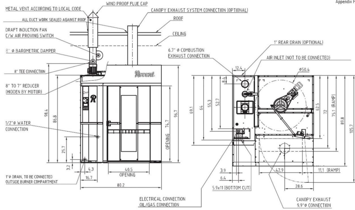
724U/SM22 OIL/GAS 700-SERIES CANOPY 701032 A
